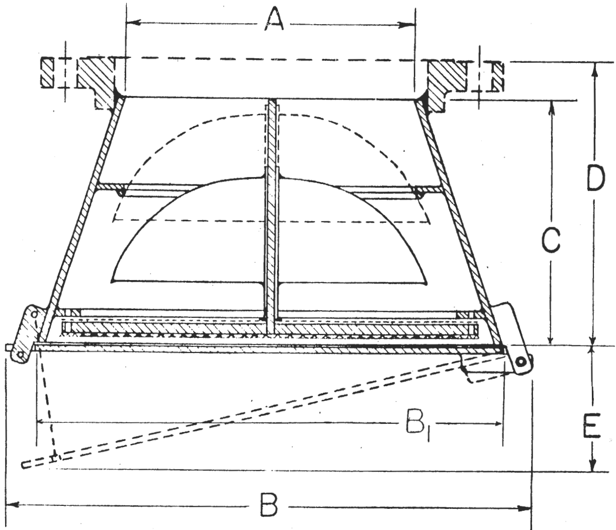
Dimensions -- Inches
