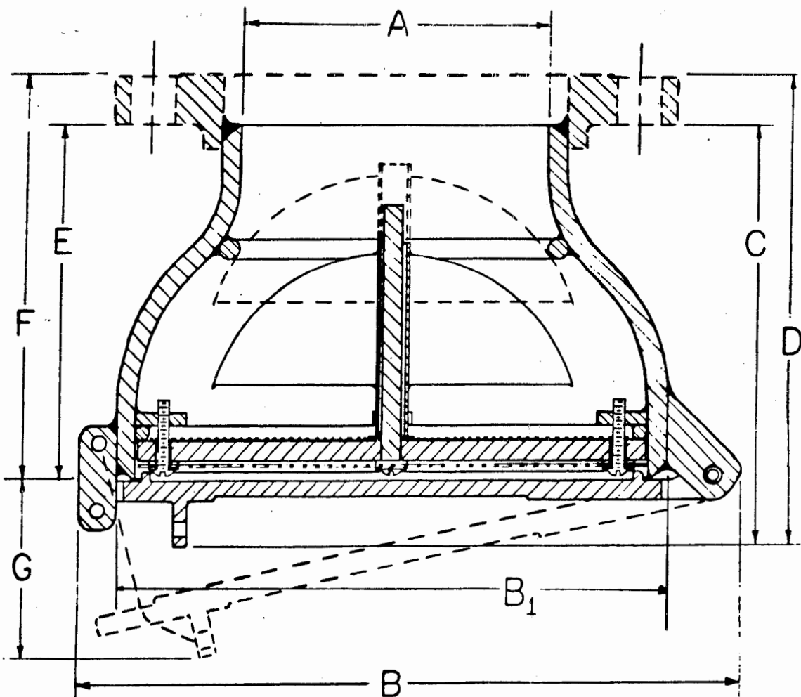
Dimensions -- Inches
